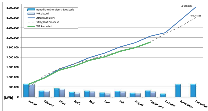
Jahresübersicht 2015 - Entwicklung der Energieerträge SL Windrad Brabecker Feld GmbH & Co. KG Windenergieanlage
