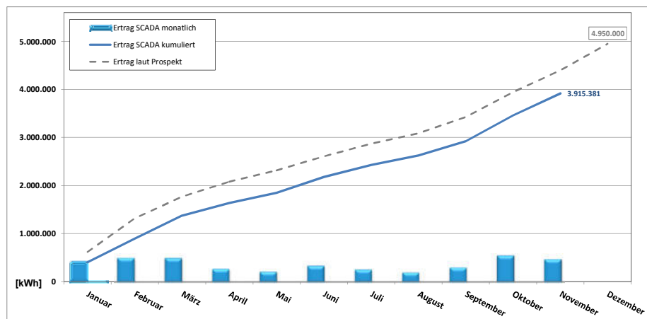
Jahresübersicht 2017 - Entwicklung der Energieerträge SL Windpark Wesel GmbH & Co. KG - E-92
