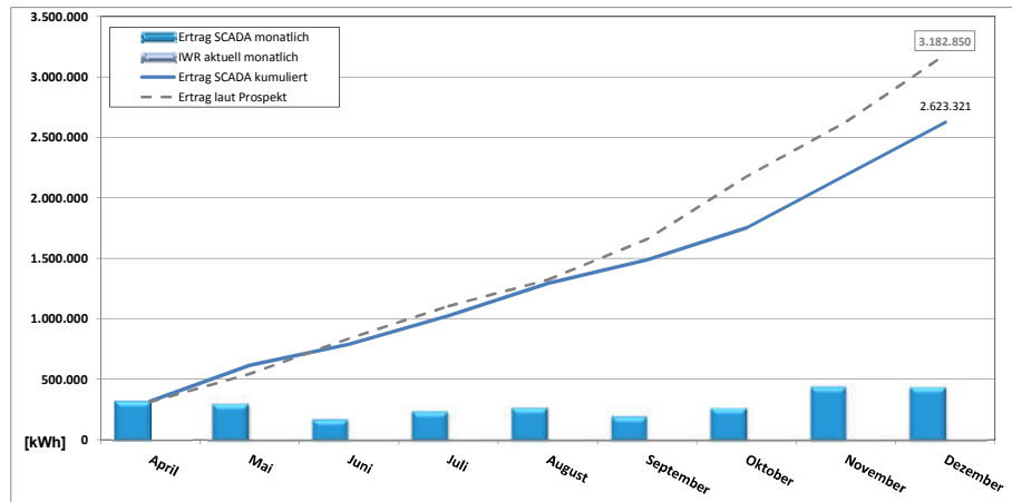
Jahresübersicht 2016 - Entwicklung der Energieerträge SL Windpark Wesel GmbH & Co. KG - E-92
