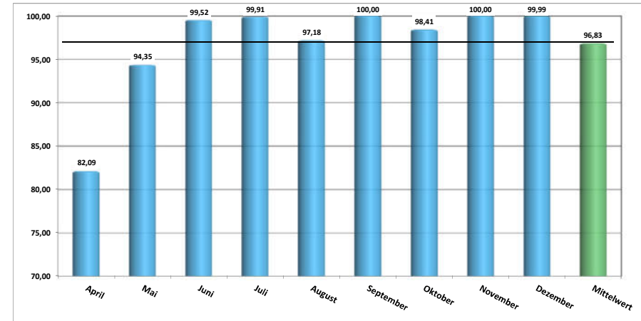
Jahresübersicht 2016 - Technische Verfügbarkeit in [%] - E-92
