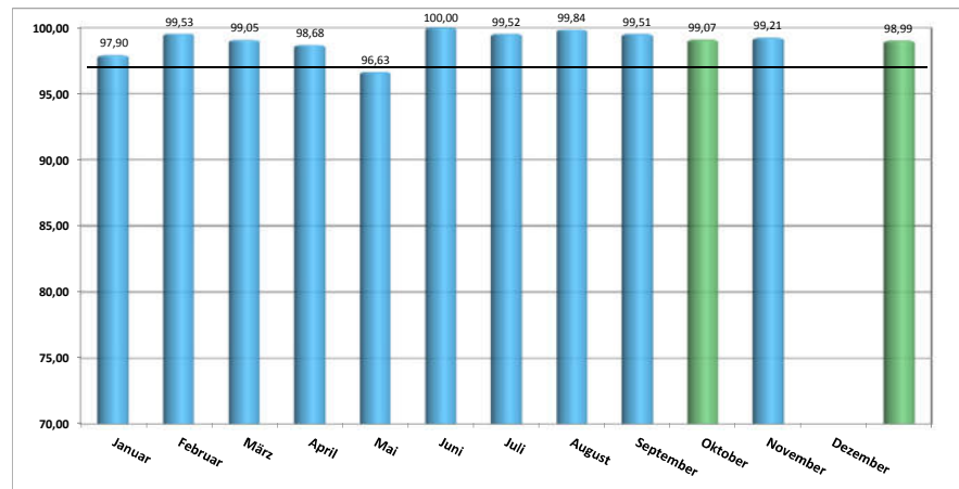
Jahresübersicht 2017 - Technische Verfügbarkeit in [%] - E-92
