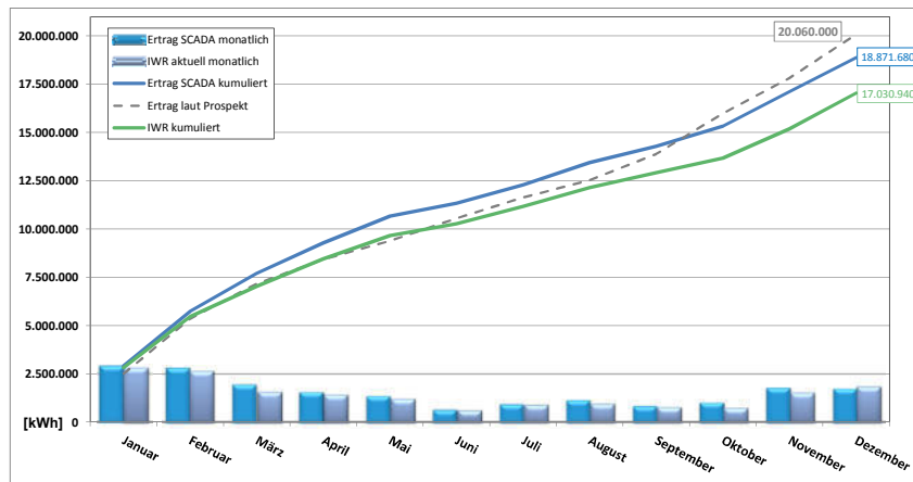
Jahresübersicht 2016 - Entwicklung der Energieerträge SL Windpark Rheurdt GmbH & Co. KG
