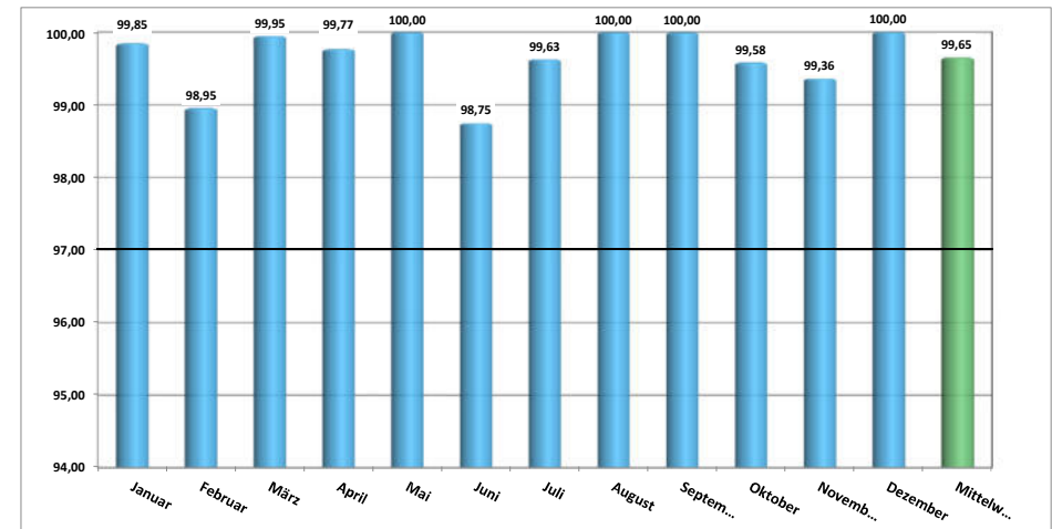
Jahresübersicht 2016 - Technische Verfügbarkeit in [%]
