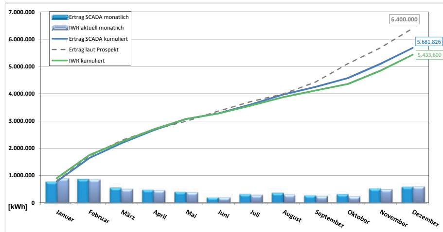
Jahresübersicht 2016 - Entwicklung der Energieerträge SL Windpark Recklinghausen GmbH & Co. KG
