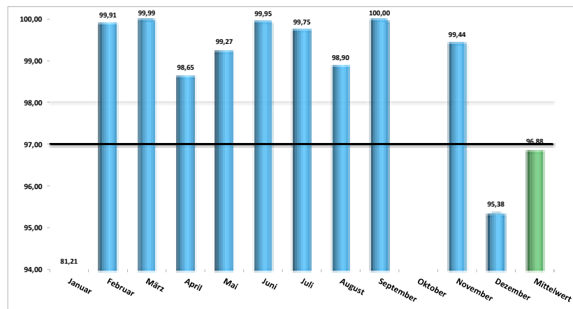
Jahresübersicht 2015 - Technische Verfügbarkeit in [%] Windenergieanlage
