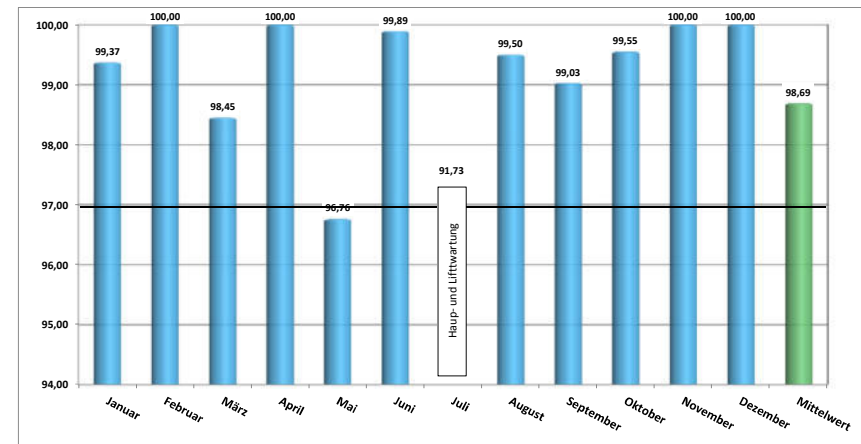
Jahresübersicht 2016 - Technische Verfügbarkeit in [%] Windenergieanlage
