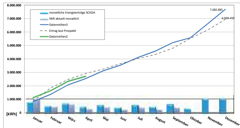
Jahresübersicht 2015 - Entwicklung der Energieerträge SL Windrad Marl GmbH & Co. KG Windenergieanlage
