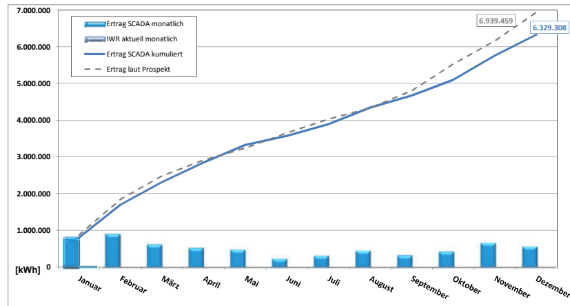
Jahresübersicht 2016 - Entwicklung der Energieerträge SL Windrad Marl GmbH & Co. KG
