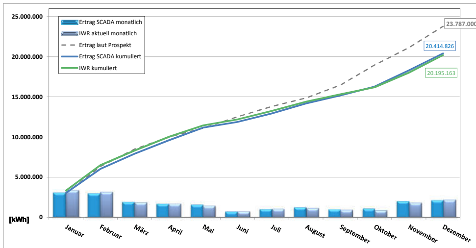
Jahresübersicht 2016 - Entwicklung der Energieerträge SL Windpark Baumberge GmbH & Co. KG
