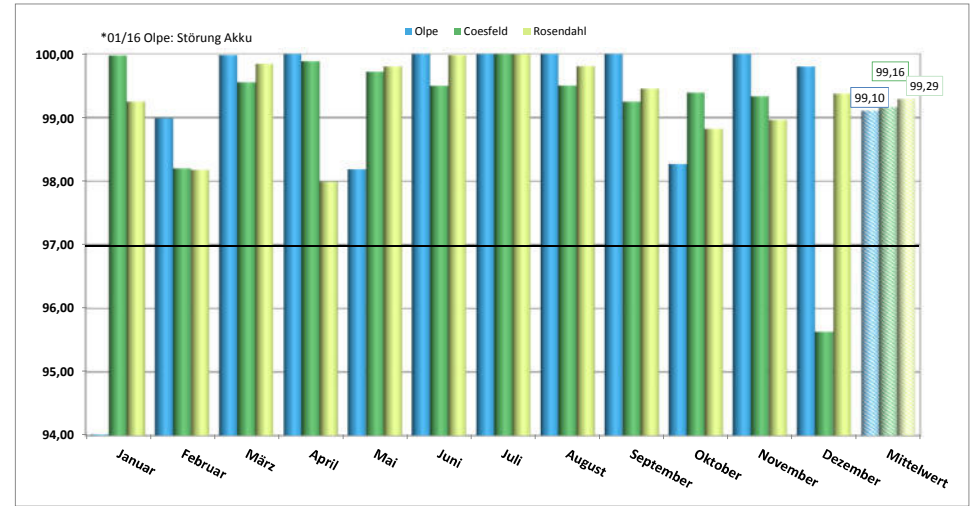
Jahresübersicht 2016 - Technische Verfügbarkeit in [%]
