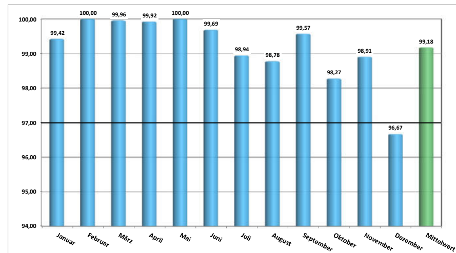
Jahresübersicht 2016 - Technische Verfügbarkeit in [%]
