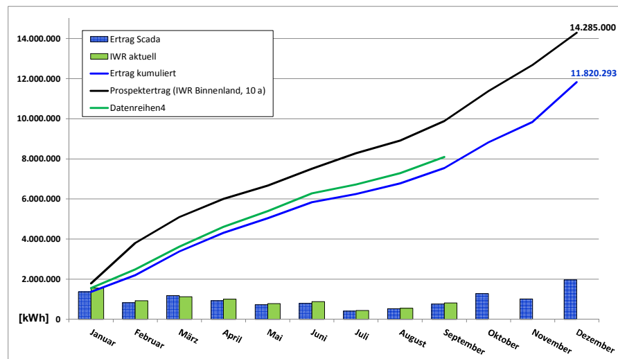
Jahresübersicht 2013 - Entwicklung der Energieerträge SL Windpark Selm GmbH & Co. KG
