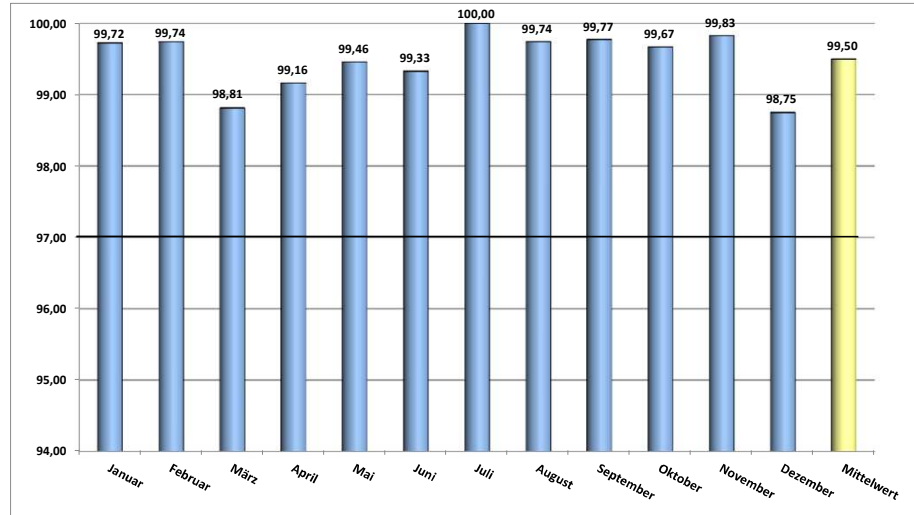
Jahresübersicht 2013 - Technische Verfügbarkeit in [%]
