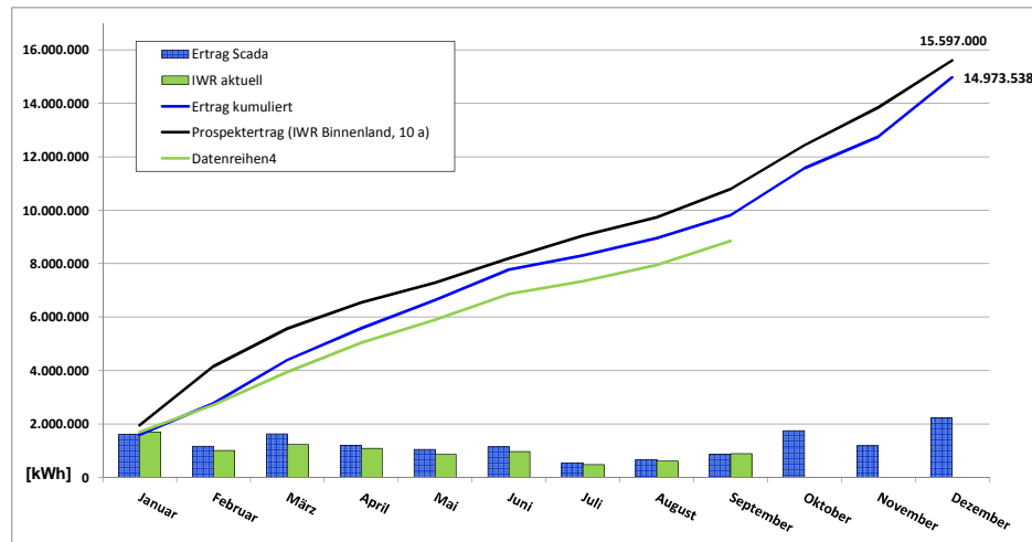
Jahresübersicht 2013 - Entwicklung der Energieerträge SL Windpark Issum GmbH & Co. KG
