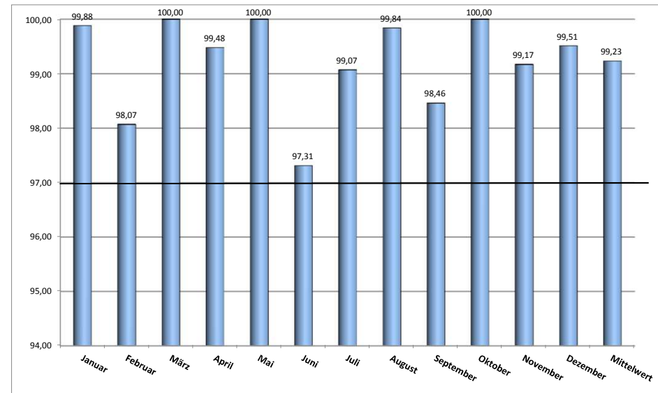
Jahresübersicht 2013 - Technische Verfügbarkeit in [%] Windenergieanlage
