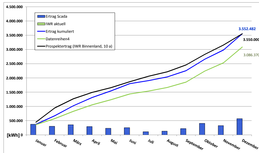
Jahresübersicht 2013 - Entwicklung der Energieerträge SL Bürgerenergie Gladbeck GmbH & Co. KG Windenergieanlage
