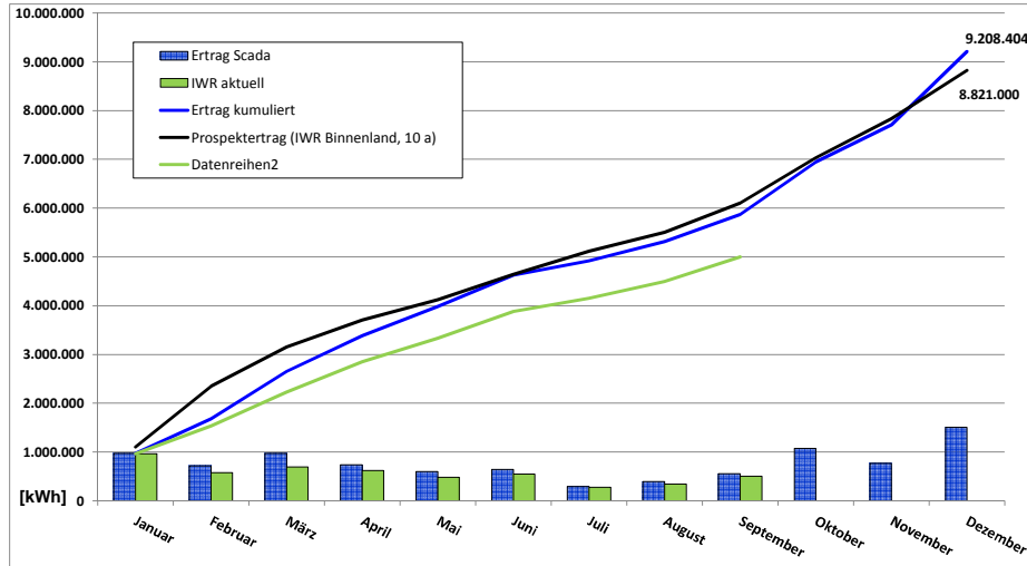
Jahresübersicht 2013 - Entwicklung der Energieerträge SL Windpark Alpen-Veen GmbH & Co. KG
