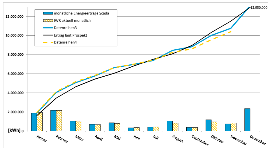
Jahresübersicht 2014 - Entwicklung der Energieerträge SL Windpark Werl GmbH & Co. KG
