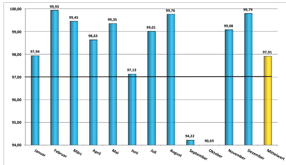
Jahresübersicht 2014 - Technische Verfügbarkeit in [%]
