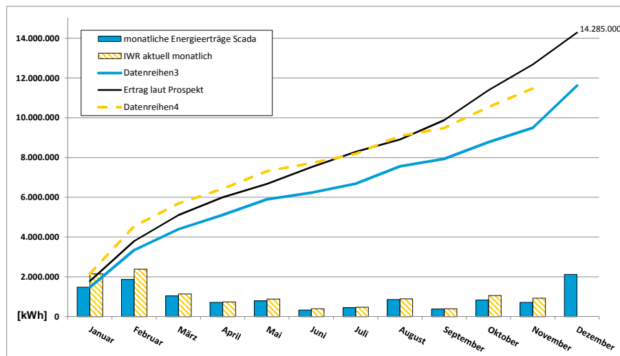
Jahresübersicht 2014 - Entwicklung der Energieerträge SL Windpark Selm GmbH & Co. KG
