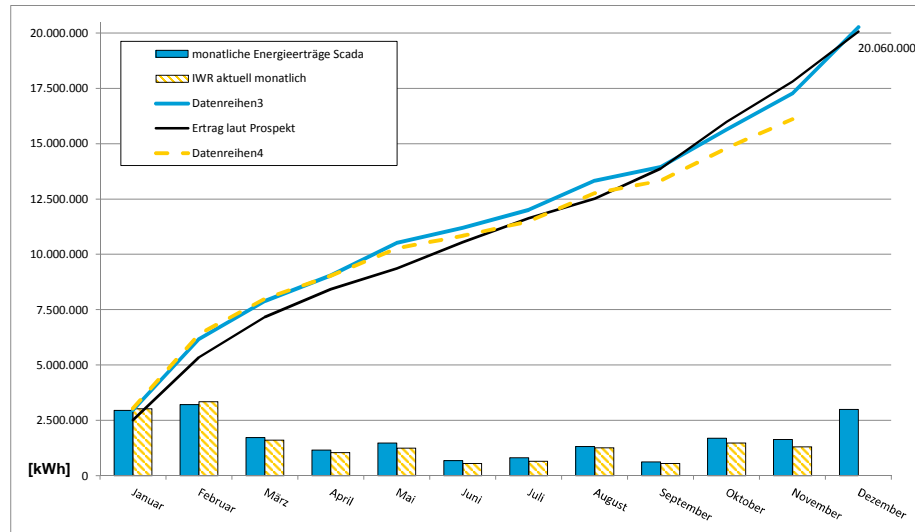
Jahresübersicht 2014 - Entwicklung der Energieerträge SL Windpark Rheurdt GmbH & Co. KG
