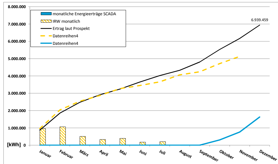
Jahresübersicht 2014 - Entwicklung der Energieerträge SL Windrad Marl GmbH & Co. KG Windenergieanlage
