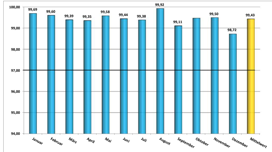
Jahresübersicht 2014 - Technische Verfügbarkeit in [%]
