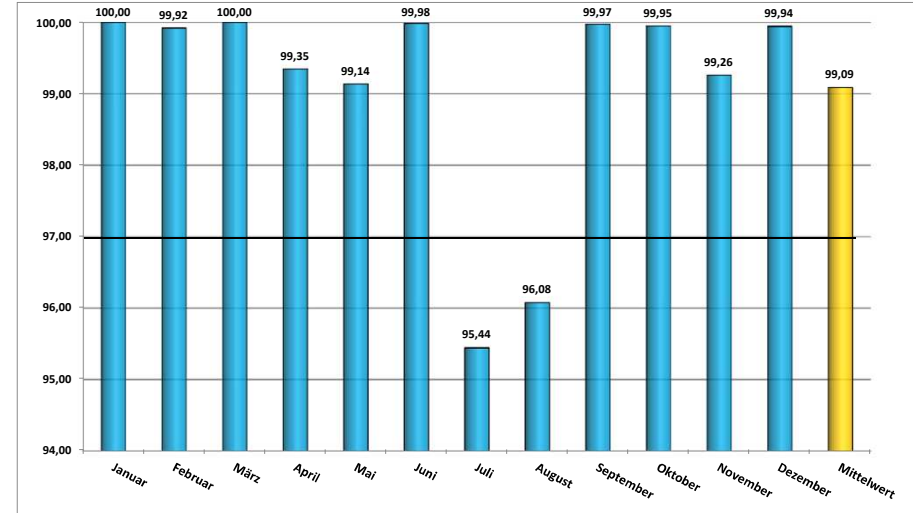
Jahresübersicht 2014 - Technische Verfügbarkeit in [%]
