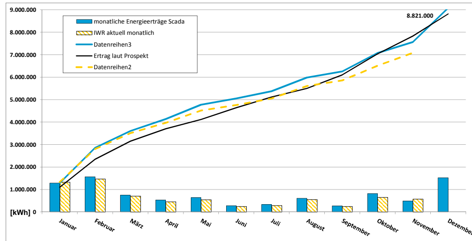
Jahresübersicht 2014 - Entwicklung der Energieerträge SL Windpark Alpen-Veen GmbH & Co. KG
