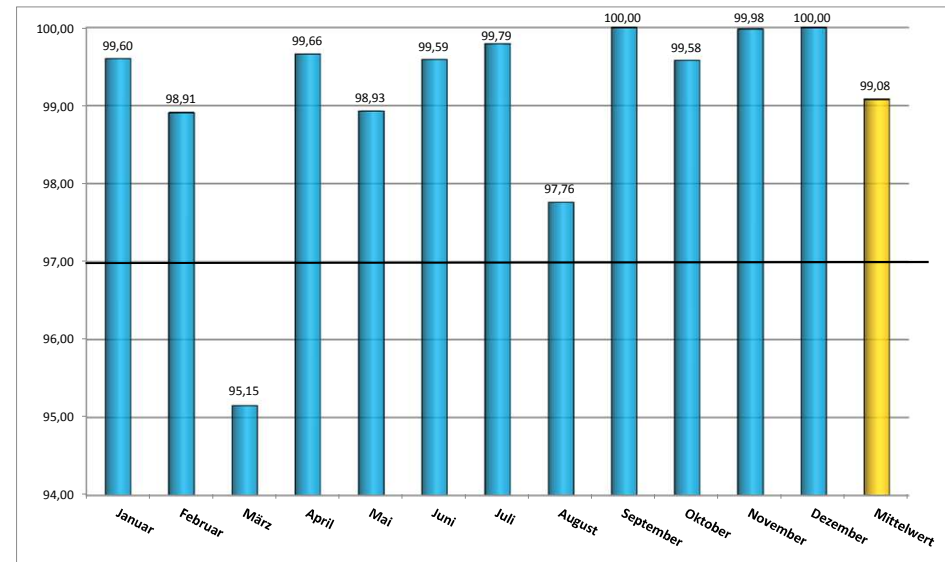
Jahresübersicht 2014 - Technische Verfügbarkeit in [%] Windenergieanlage
