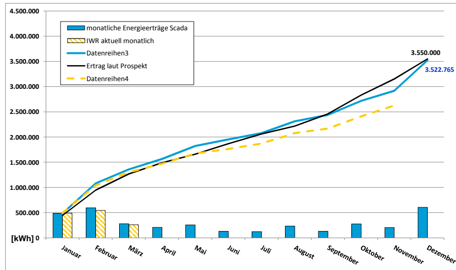
Jahresübersicht 2014 - Entwicklung der Energieerträge SL Bürgerenergie Gladbeck GmbH & Co. KG Windenergieanlage
