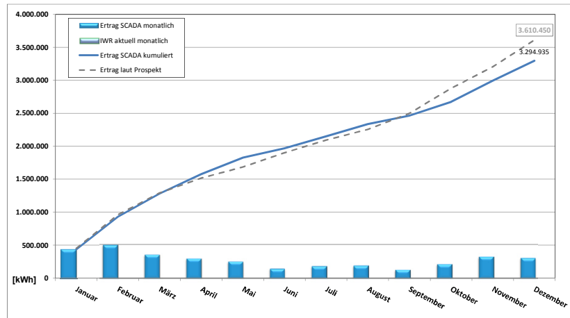
Jahresübersicht 2016 - Entwicklung der Energieerträge SL Windrad Wiesenbusch GmbH & Co. KG
