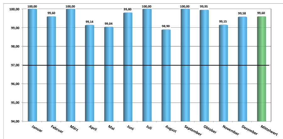
Jahresübersicht 2016 - Technische Verfügbarkeit in [%] Windenergieanlage
