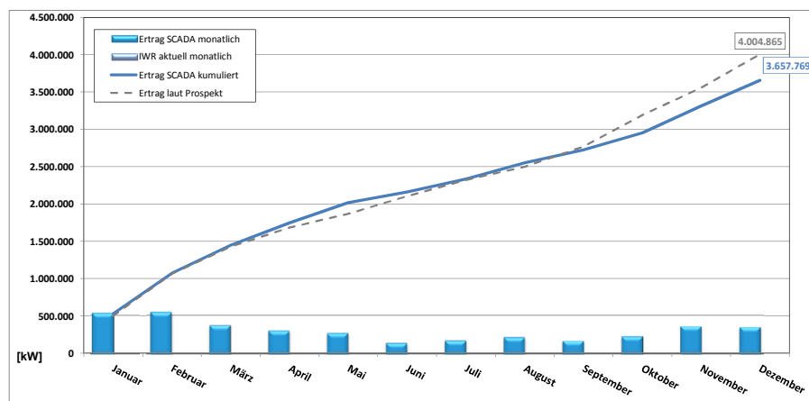
Jahresübersicht 2016 - Entwicklung der Energieerträge SL Windrad Brabecker Feld GmbH & Co. KG
