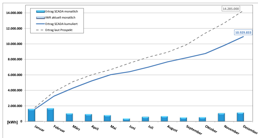
Jahresübersicht 2016 - Entwicklung der Energieerträge SL Windpark Selm GmbH & Co. KG
