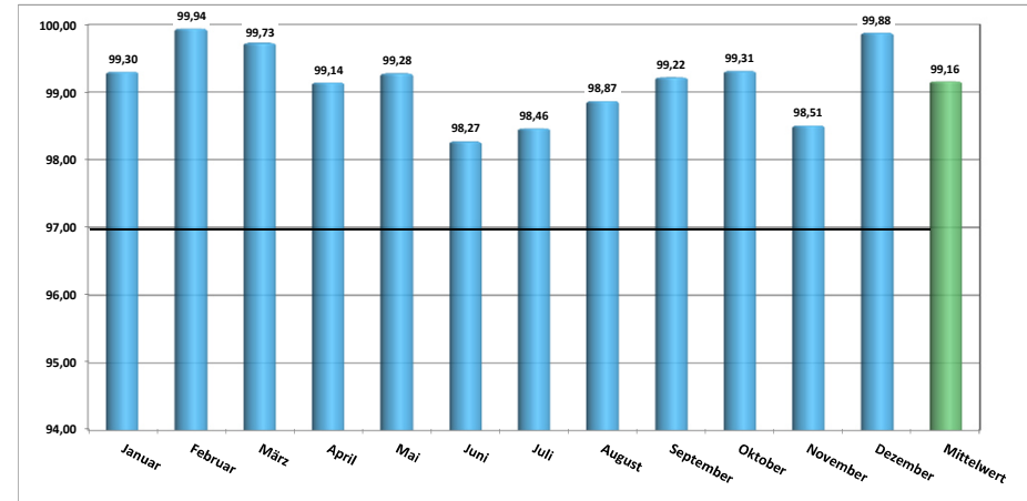
Jahresübersicht 2016 - Technische Verfügbarkeit in [%]
