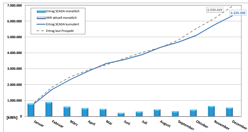
Jahresübersicht 2016 - Entwicklung der Energieerträge SL Windrad Marl GmbH & Co. KG
