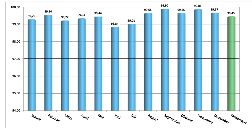
Jahresübersicht 2016 - Technische Verfügbarkeit in [%]
