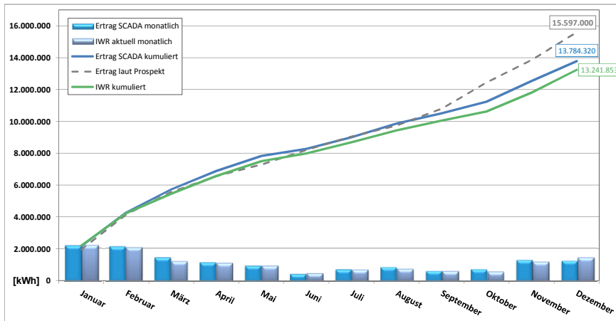
Jahresübersicht 2016 - Entwicklung der Energieerträge SL Windpark Issum GmbH & Co. KG
