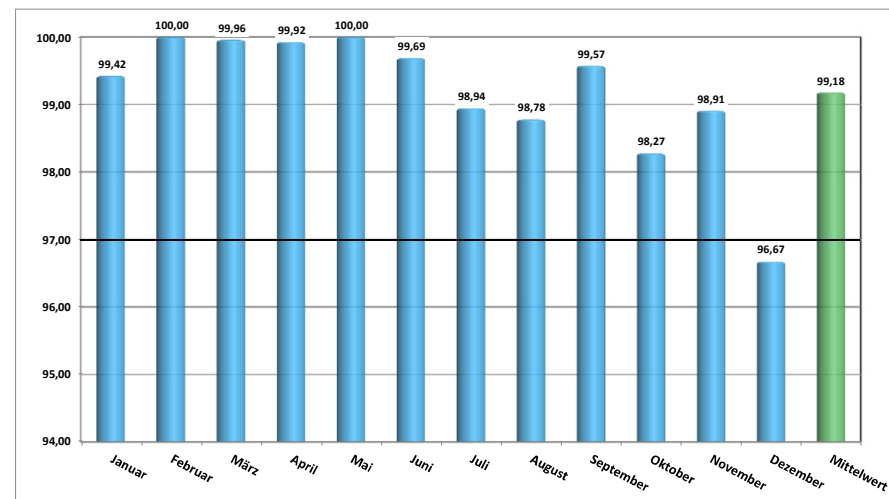
Jahresübersicht 2016 - Technische Verfügbarkeit in [%]
