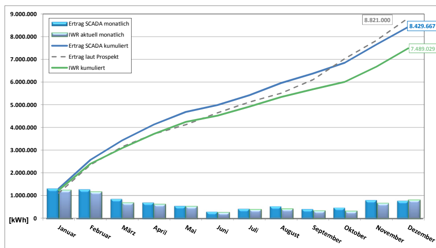
Jahresübersicht 2016 - Entwicklung der Energieerträge SL Windpark Alpen-Veen GmbH & Co. KG
