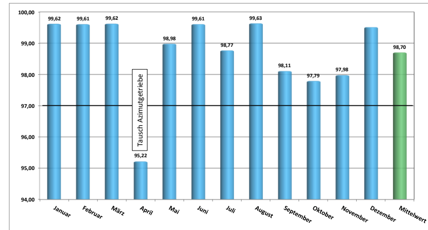
Jahresübersicht 2015 - Technische Verfügbarkeit in [%]
