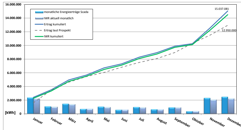
Jahresübersicht 2015 - Entwicklung der Energieerträge SL Windpark Werl GmbH & Co. KG
