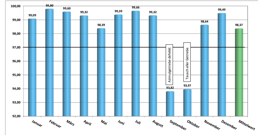
Jahresübersicht 2015 - Technische Verfügbarkeit in [%]
