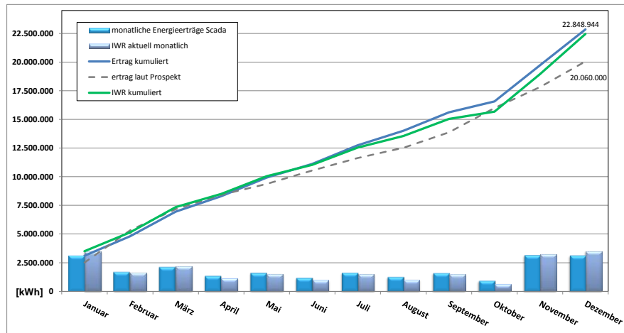
Jahresübersicht 2015 - Entwicklung der Energieerträge SL Windpark Rheurdt GmbH & Co. KG
