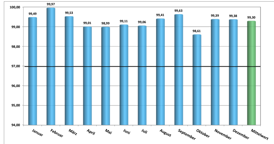
Jahresübersicht 2015 - Technische Verfügbarkeit in [%]
