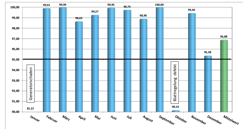
Jahresübersicht 2015 - Technische Verfügbarkeit in [%] Windenergieanlage
