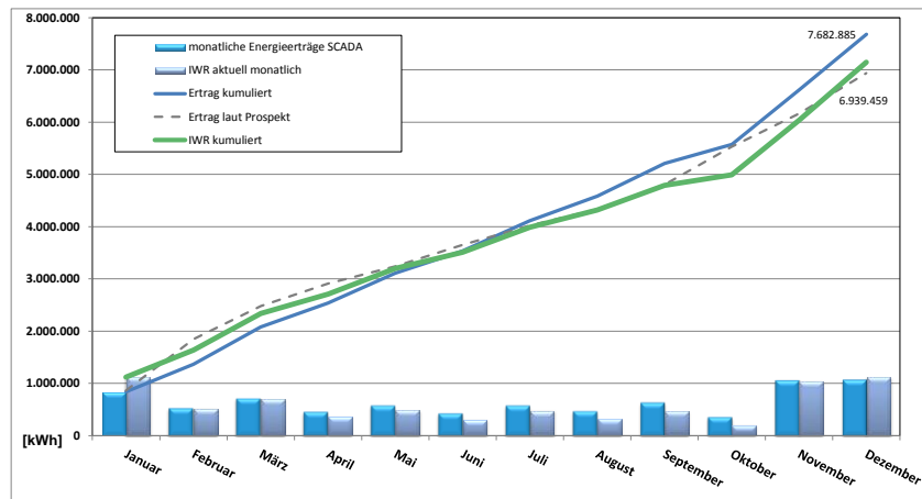
Jahresübersicht 2015 - Entwicklung der Energieerträge SL Windrad Marl GmbH & Co. KG
